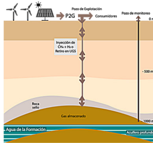
Figura 7. Esquema general de los elementos de un AGH en un acuífero salino profundo. (P. G. Haddad, 2022).
