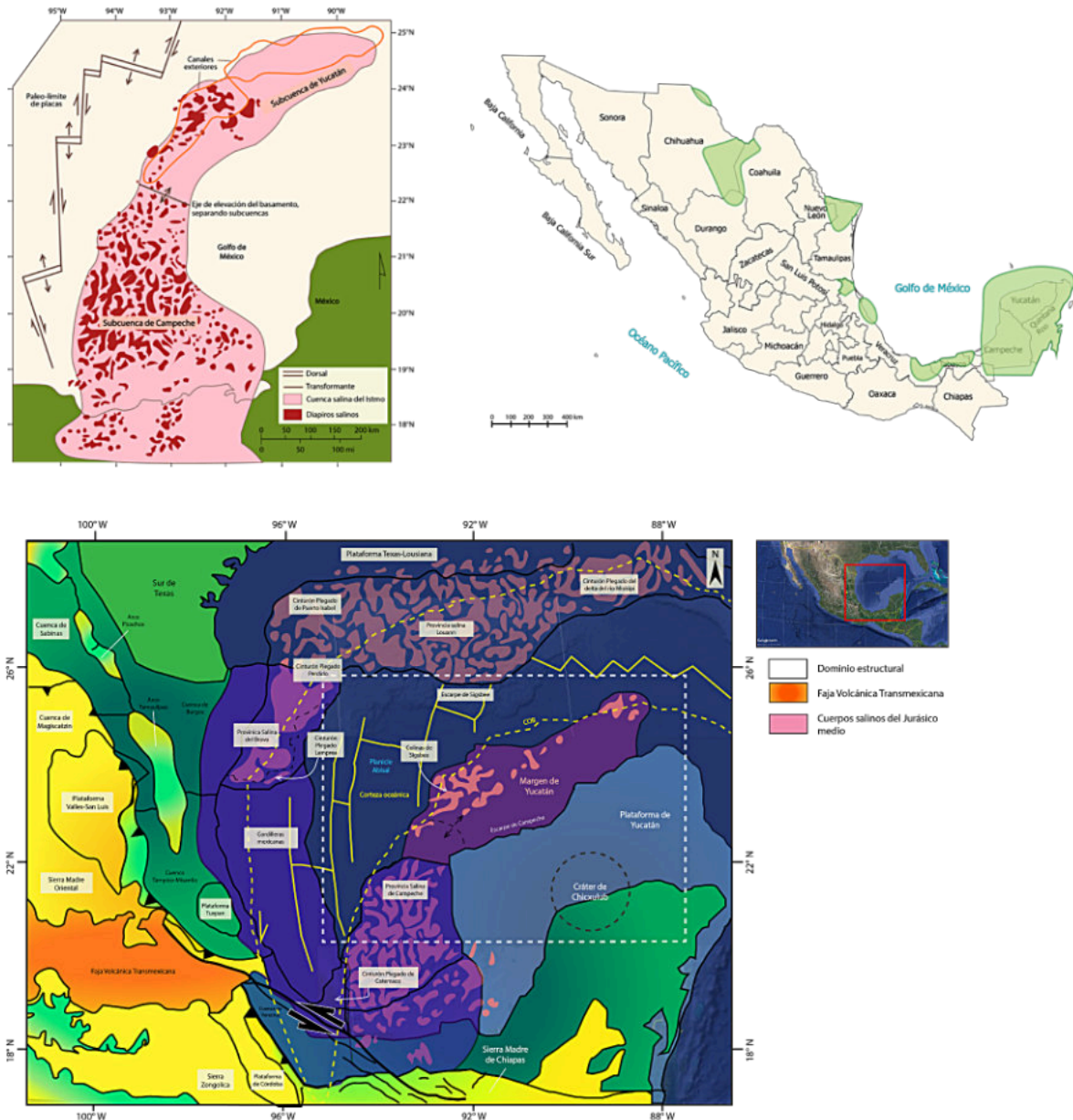
Figura 22 . Regiones con estructuras salinas en México y detalle en la cuenca salina del sureste. Modificado de (Kenning J. J., 2020) y (Hernández Mendoza, 2007).
