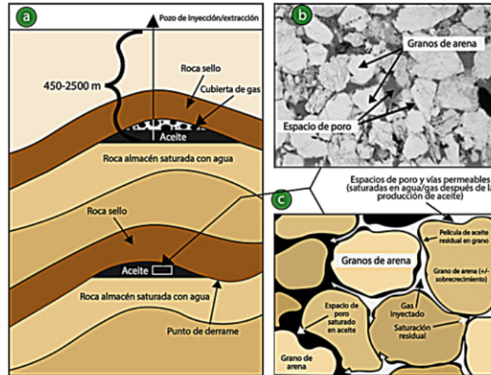
Figura 6. Condición general de un yacimiento exhausto de hidrocarburo (a); imagen microscópica de los poros con hidrocarburo (b), y cuando el H 2 evacua parcialmente el hidrocarburo remanente de los poros (c). (Nasiru Salahu Muhammeda, 2022).
