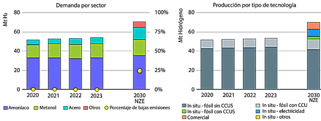
Figura 16. Uso del H 2 en el sector industrial y proyección al 2030, histórica y en escenario net-cero. (IEA, 2024).
